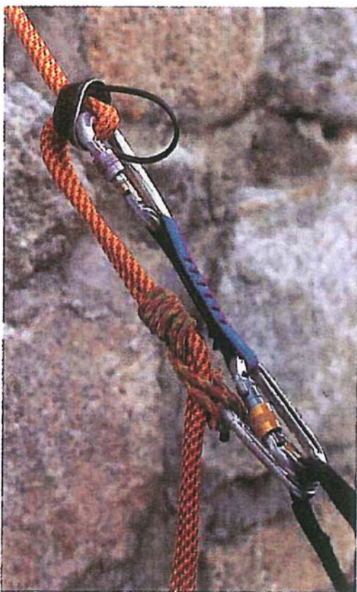
Slaňovací oko úvazku
