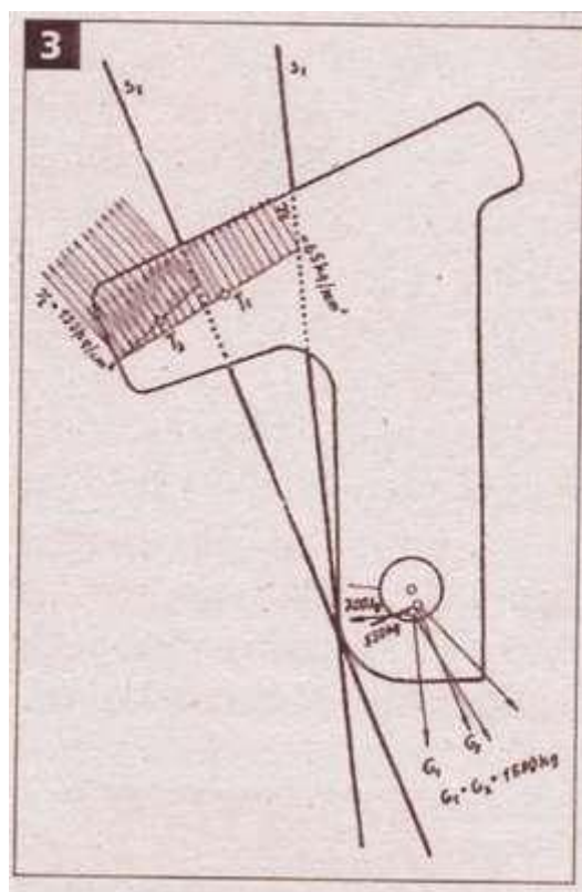
Nákres Šádkovy jedničky z článku ing. Mazáčka, Šádkova technologia, časopis Turistika a horolezectví 1952
